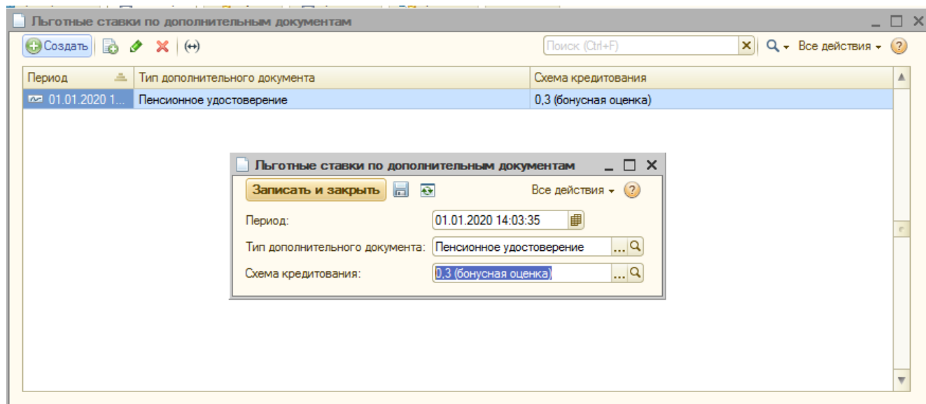
Рис. 5.10 Форма редактирования регистра « Льготные ставки по дополнительным документам ».
