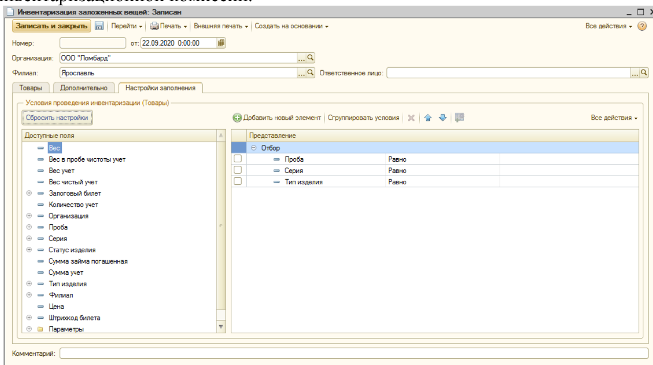
Рис. 3.11. Инвентаризация заложенных вещей. Настройки заполнения.
